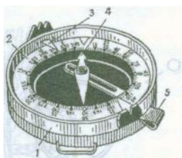
Рис. 133. Компас Адрианова: 1 — крышка со стойками для визирования; 2 — лимб; 3 — указатель отсчета; 4 — магнитная стрелка; 5 — тормоз.
